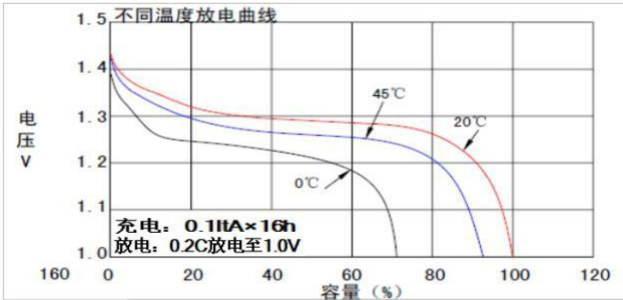
特征曲线
