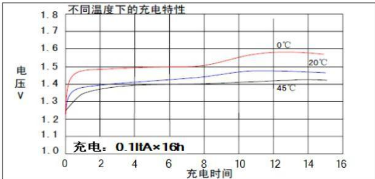
特征曲线
